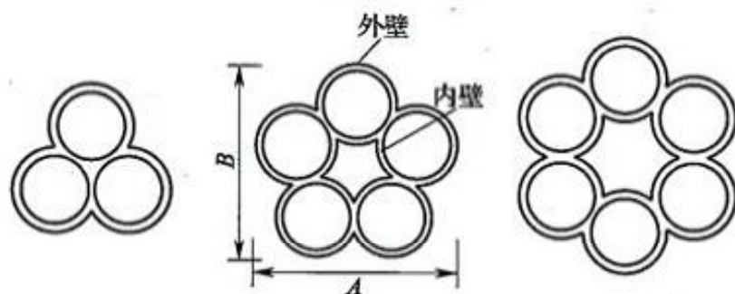
图7 梅花式塑料管横断面形式
