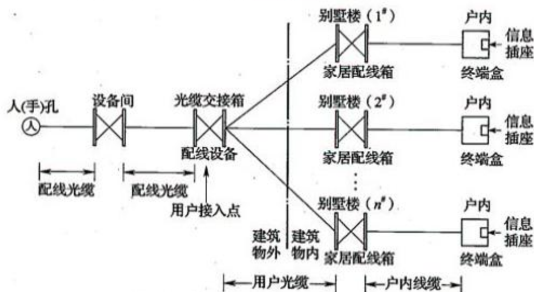
图 4 别墅建筑用户接入点设置示意
