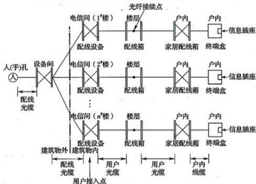
图 2 高层住宅建筑用户接入点位置示意
