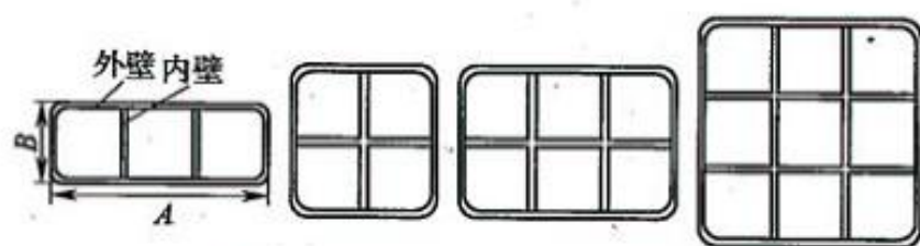
图5 栅格式塑料管横断面形式
